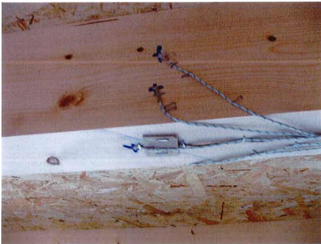
Vues de détails des solives du plancher de référence et de l'instrumentation des solives
