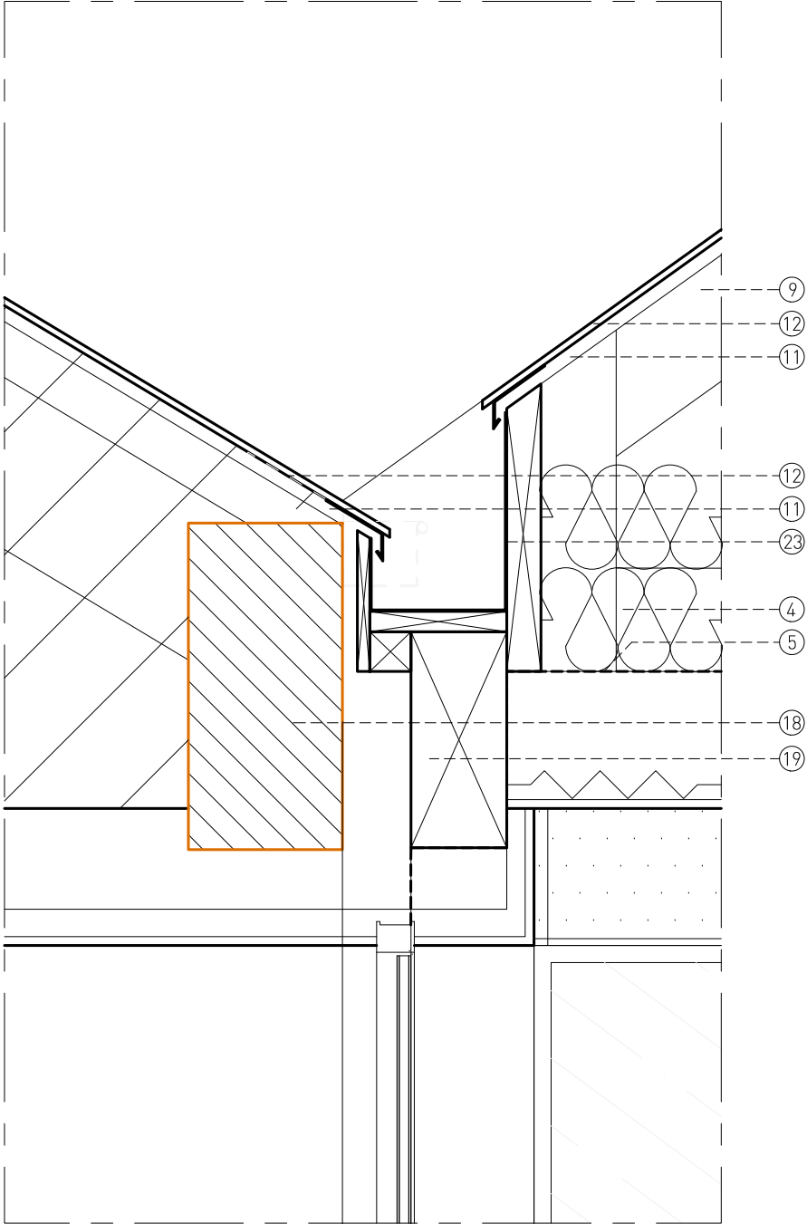
DETAIL CHENEAU EN LINTEAU I I/10
