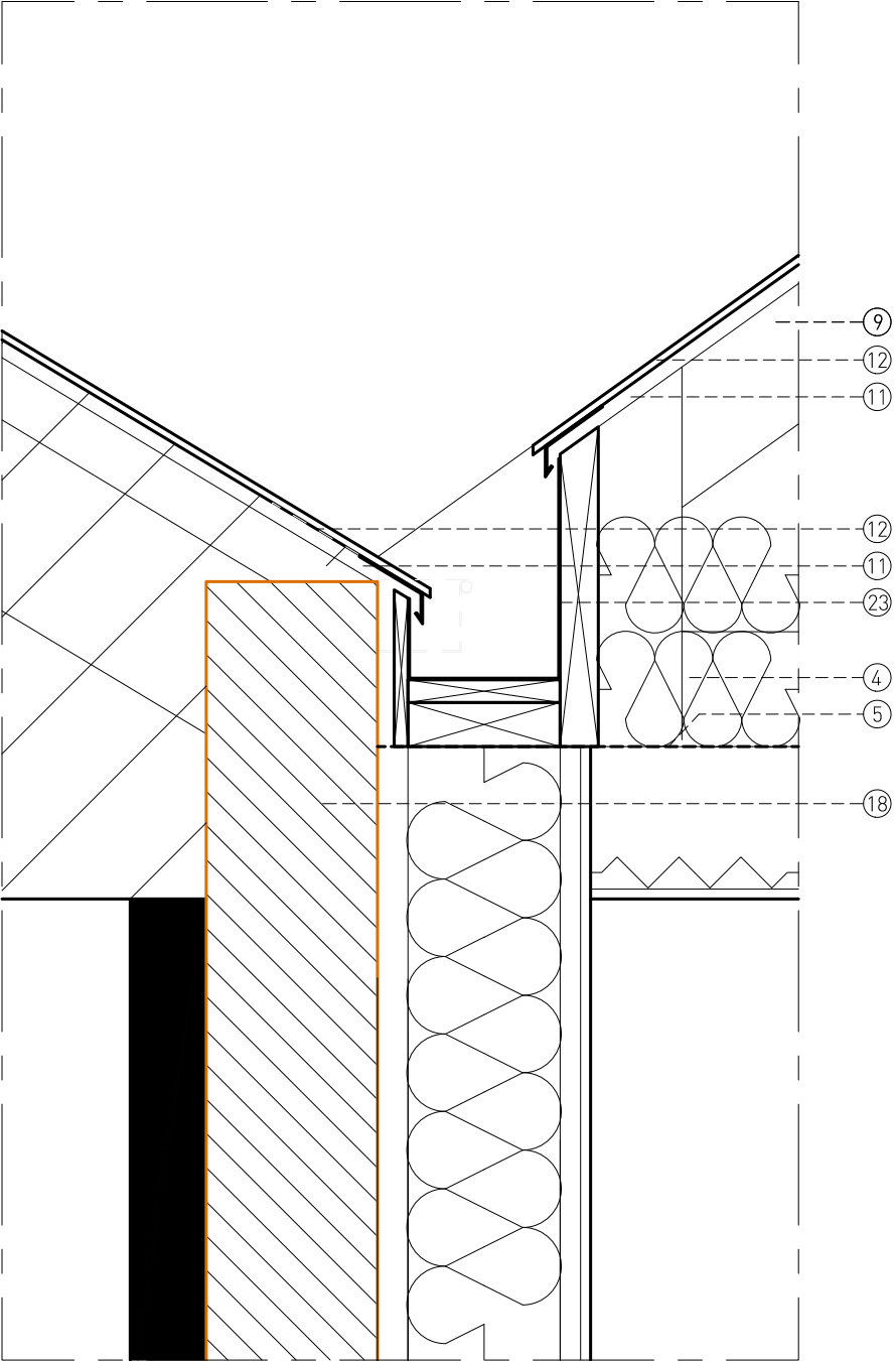
DETAIL CHENEAU EN MOB RAJOUTE I I/10
