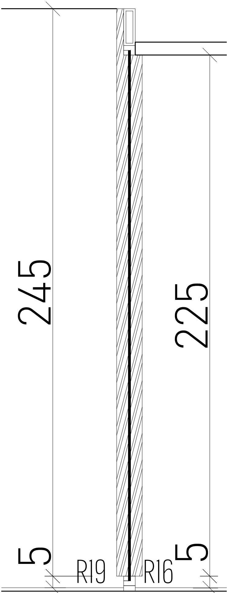
DETAIL PAROI VITREE AVEC BRISES VUE BOIS ENTRE R16 et R19 I I/10
