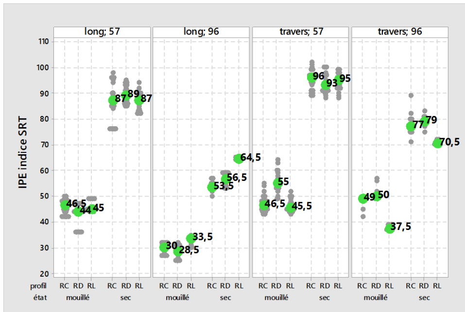
Figure 16 Résultats d'essais pendue SRT selon NF EN 16165 annexe C sur lames Ipé profil Lisse, profil RC, profil RD, sec et mouillé, avec le patin 57 puis avec le patin 96, en sens long puis en sens travers.
