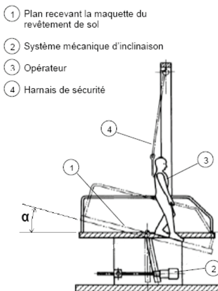
Figure 4 Principe essais plan incliné selon NF EN 16165 annexe A et B
