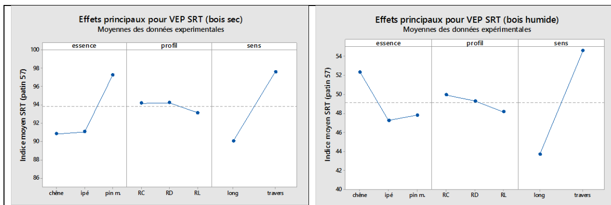
Figure 14 Effets principaux sur bois sec et sur bois humide
