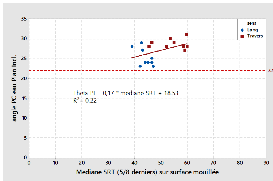
Figure 19 Recherche de corrélation entre l'essai plan incliné avec polluant de type eau selon NF EN 16165 annexe A adapté, et essai pendule SRT avec polluant de type eau selon NF EN 16165 annexe C. Les résultats sens long et les résultats sens travers considérés ensemble
