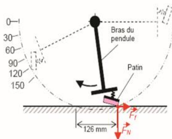
Figure 9 Principe essais pendule SRT selon NF EN 16165 annexe C
