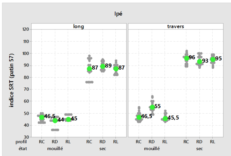
Figure 13 Résultats d'essais pendule SRT selon NF EN 16165 annexe C sur lames Ipé Lisse, profil RC, profil RD, sec et mouillé en sens long puis en sens travers
