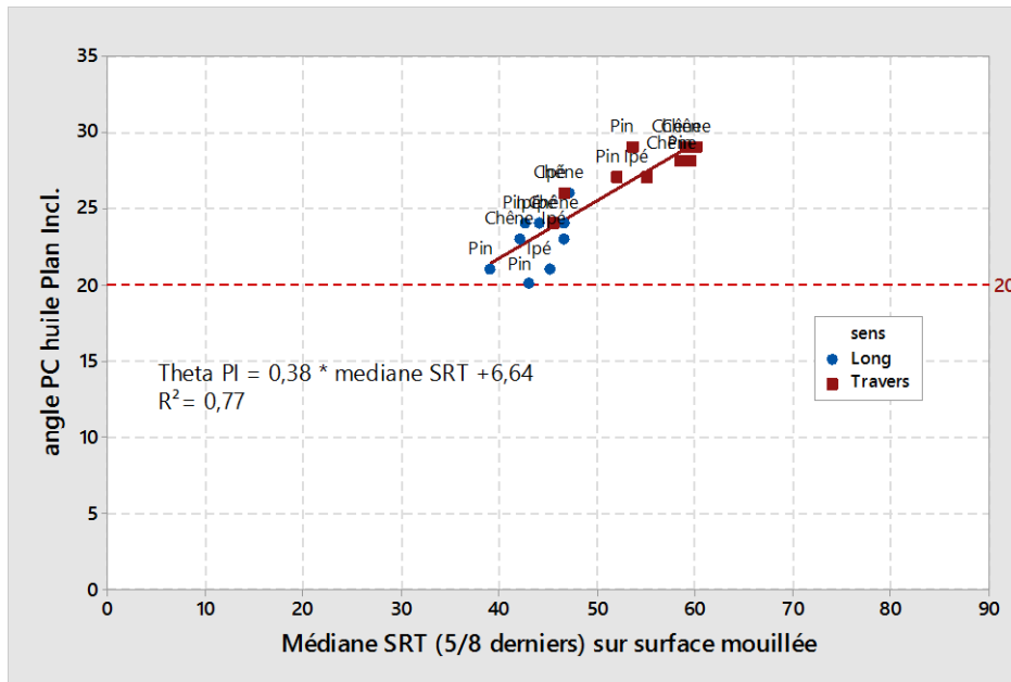
Figure 18 Recherche de corrélation entre l'essai plan incliné avec polluant de type huile selon NF EN 16165 annexe B et essai pendule SRT avec polluant de type eau selon NF EN 16165 annexe C. Les résultats sens long et les résultats sens travers considérés ensemble
