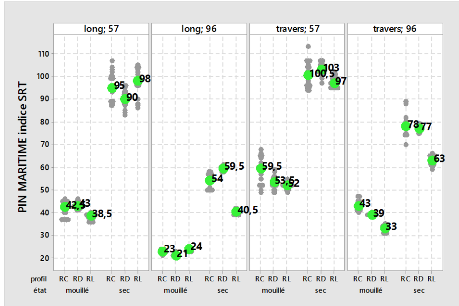
Figure 15 Résultats d'essais pendue SRT selon NF EN 16165 annexe C sur lames Pin profil Lisse, profil RC, profil RD, sec et mouillé, avec le patin 57 puis avec le patin 96, en sens long puis en sens travers.
