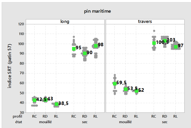
Figure 11 : Résultats d'essais pendule SRT selon NF EN 16165 annexe C sur lames Pin Lisse, profil RC, profil RD, sec et mouillé en sens long puis en sens travers
