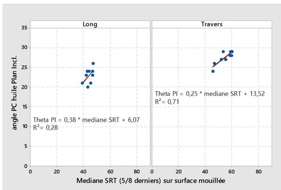
Figure 17 Recherche de corrélation entre l'essai plan incliné avec polluant de type huile selon NF EN 16165 annexe B et essai pendule SRT avec polluant de type eau selon NF EN 16165 annexe C. Les résultats sens long et les résultats sens travers considérés séparément
