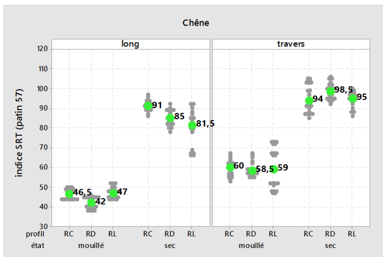
Figure 12 : Résultats d'essais pendule SRT selon NF EN 16165 annexe C sur lames Chêne Lisse, profil RC, profil RD, sec et mouillé en sens long puis en sens travers
