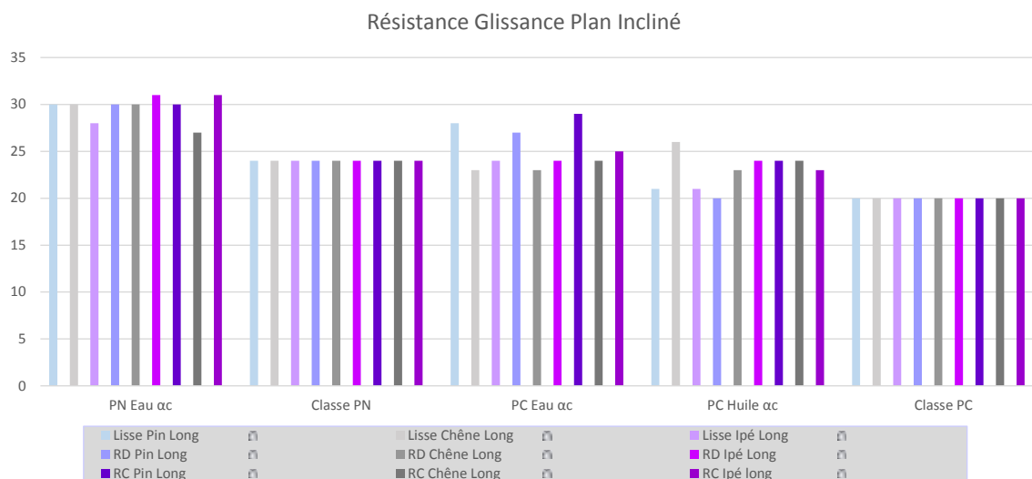
Figure 6 Résultats d'essais plan incliné sur lames Pin (teintes bleutées), lames Chêne (teintes grisées), lames Ipé (teintes violets) en sens long.
