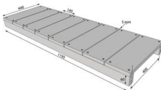
Figure 3 Maquette sens travers
