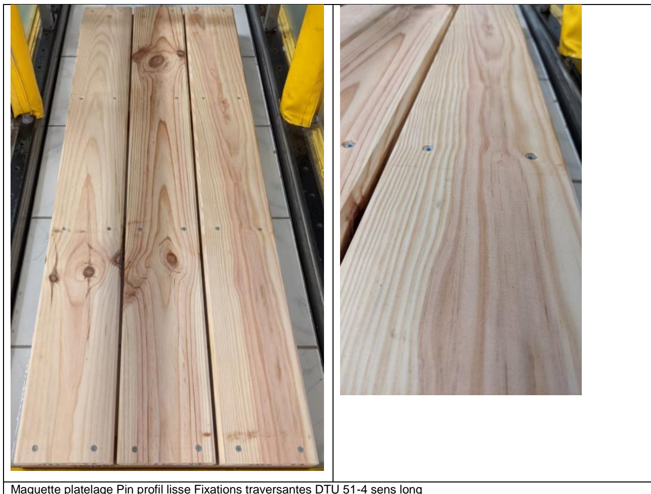
Figure 5 Photo maquettes plan incliné selon NF EN 16165 annexe A et B
