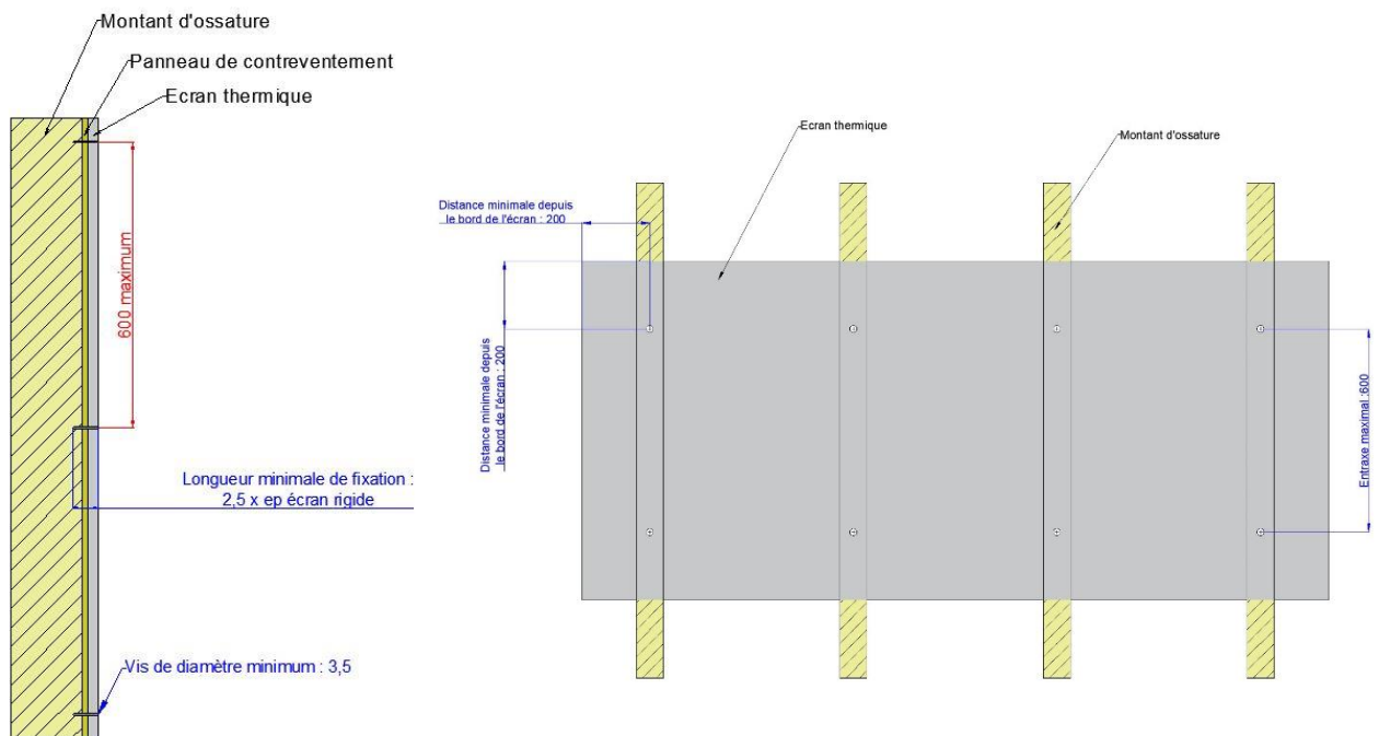
Figure 3 : Dispositions pour la fixation de l'écran thermique
