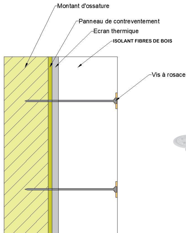
Figure 2 : Fixation de l'ETICS sur support bois avec vis à rosace
